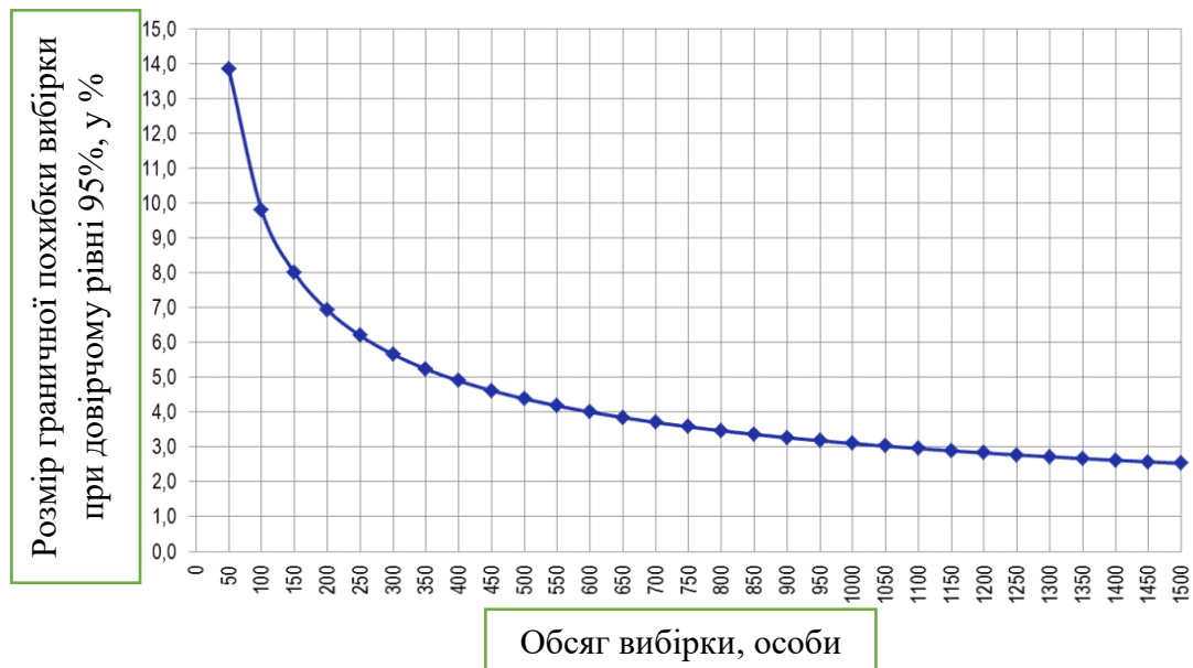
Рис. 3.1. Крива залежності граничної помилки вибірки від її обсягу [2]
